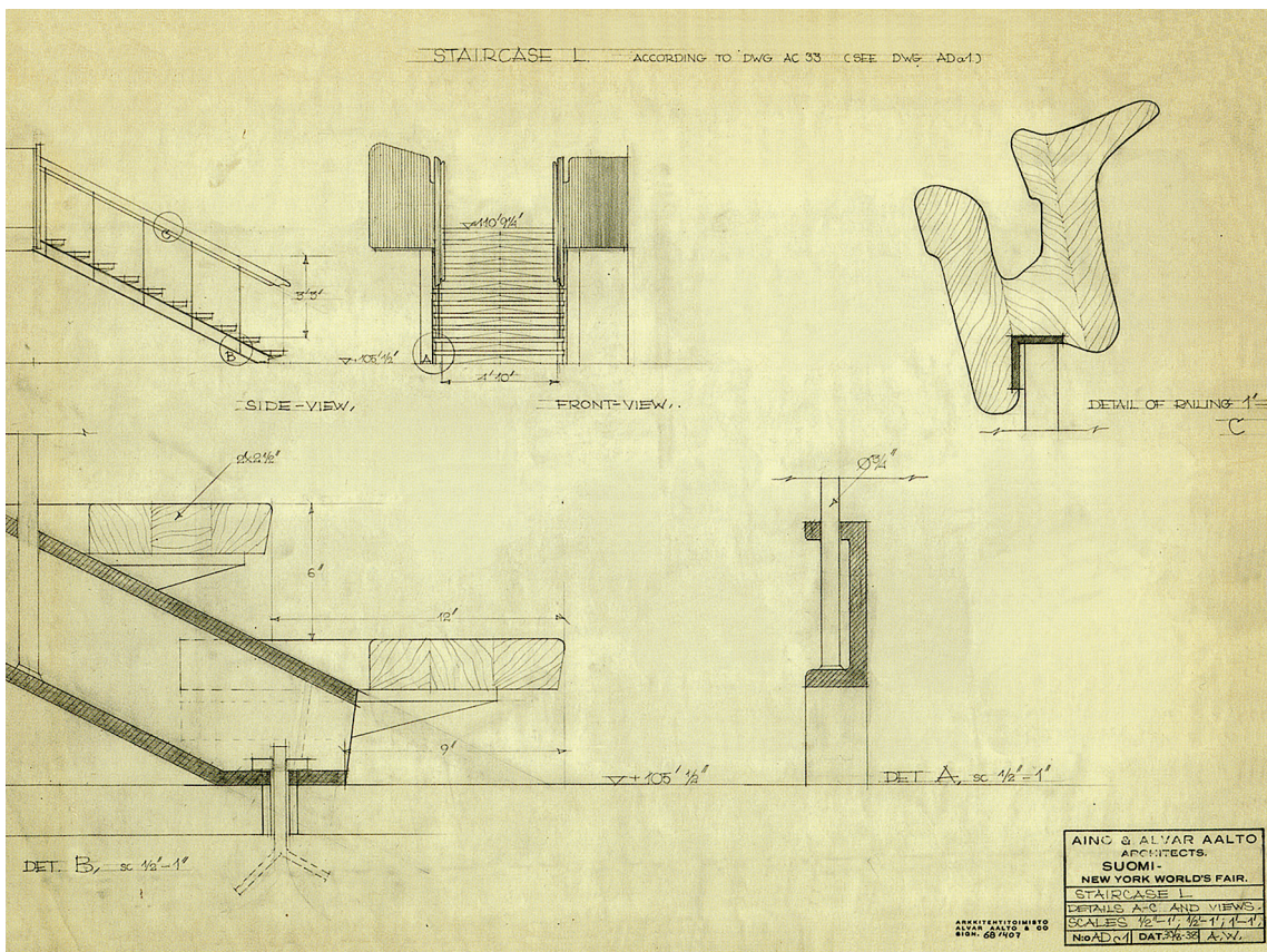
Aino ja Alvar Aallon luonnospirustuksia New Yorkin maailmannäyttelyn Suomen paviljonkia varten (1939). Julkaistu teoksessa Alvar Aalto, Puu taipuu (2010).
